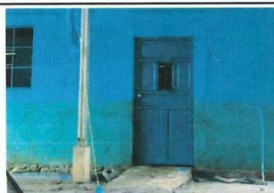
Foto 6: Sustitución e instalacion de puerta de madera por metal, 2.10 x 1 m.
